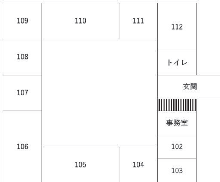
1F 平面図
