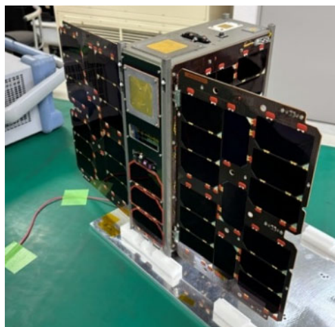
超小型衛星「VERTECS」
