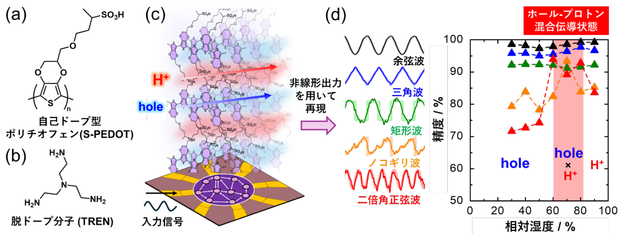
図 1. (a) 自己ドーブ型ポリチオフェン (S-PEDOT) と (b) 脱ドーブ分子である多価アミンの化学構造、 (c) 本系におけるホール-プロトン混合伝導状態を示すイメージ図。(d) 混合伝導状態を示す条件にてマテリアルリザー素子の性能 (波形生成タスクの精度) が向上することを示す図。
