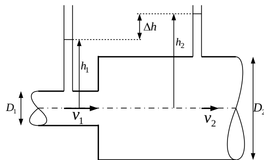
図-1 水平円管の急拡大
