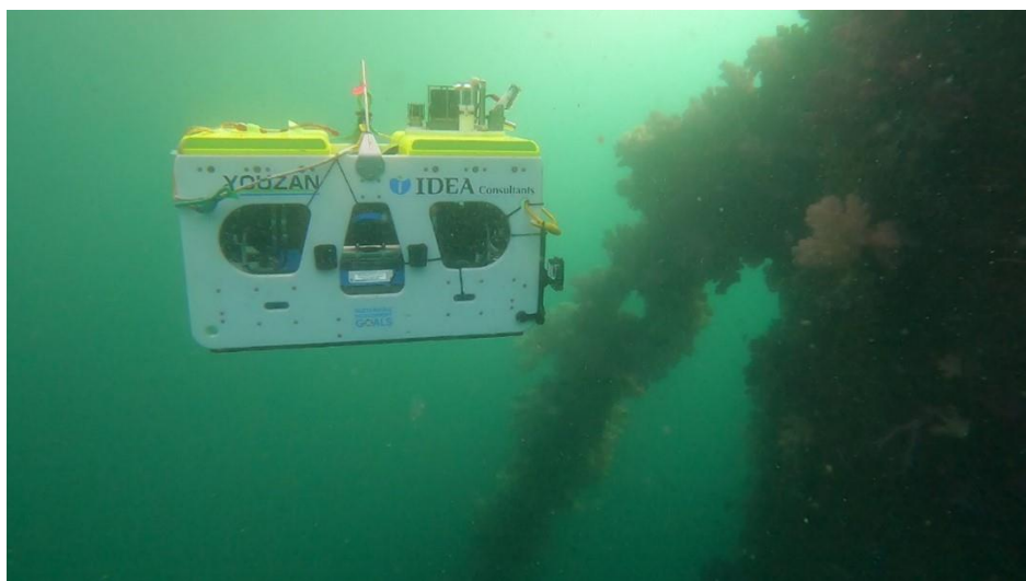
写真 3 係留チェーン接続部の回避状況
