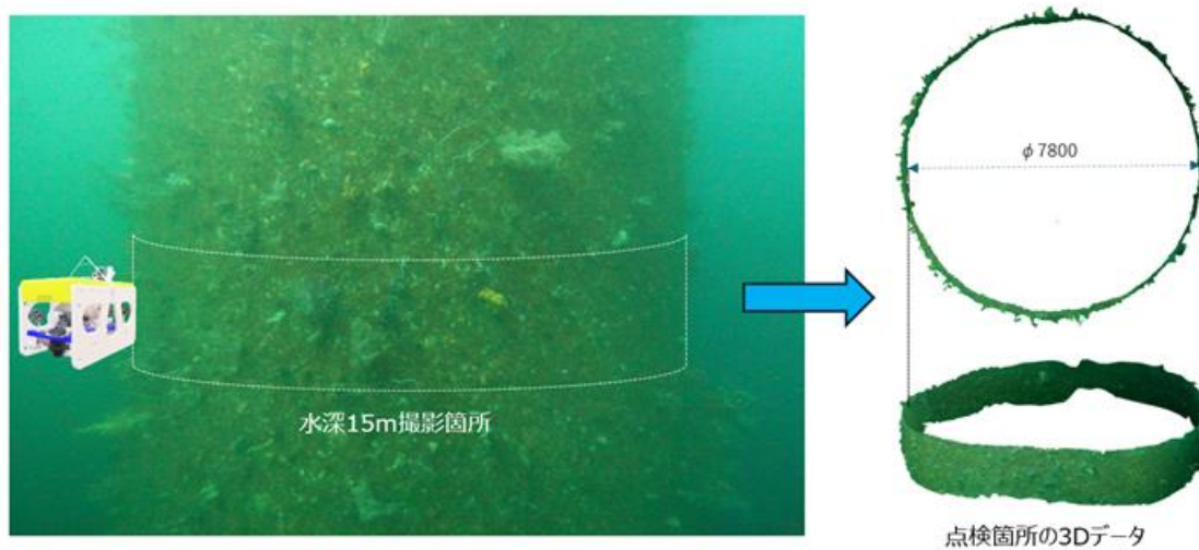
図 2 スパー型浮体の 3D データ(水深 15m)
