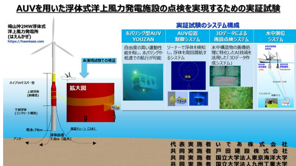
図 1 AUV を用いた浮体式洋上風力発電施設の点検を実現するための実証試験概要
