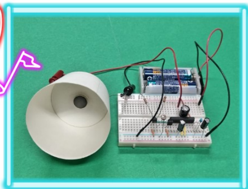
紙コップスピーカーと電子回路 (外箱は当日お渡しします)
